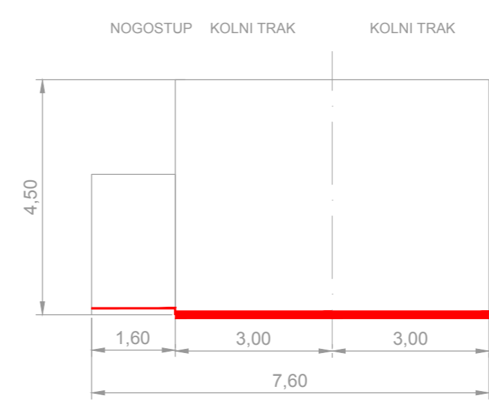
PRESJEK 1-1
