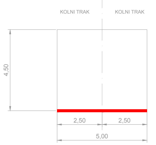
PRESJEK 2-2
